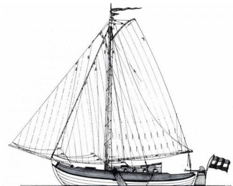
Vollenhovens Boljacht 9.75 x 3.25 / 3.45 x 0.65 m.
